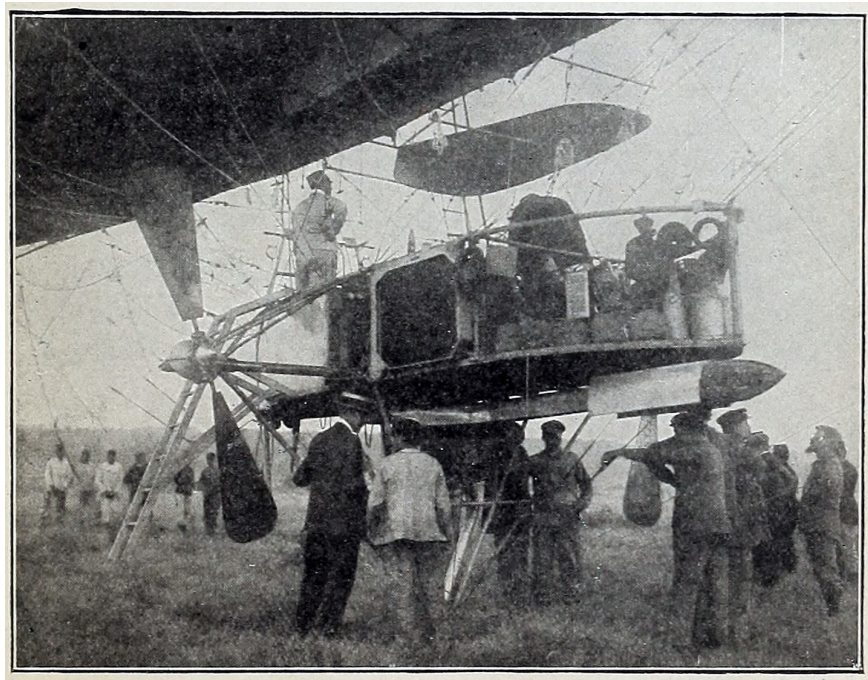
Fig. 11. Car of La Republique
