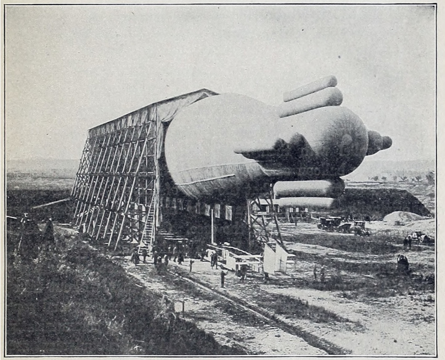
Fig. 8. La Ville de Paris Showing Balloonets
